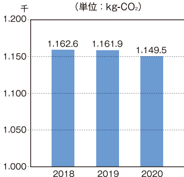
車両由来CO 2 推移 (単位: kg-CO 2 )
